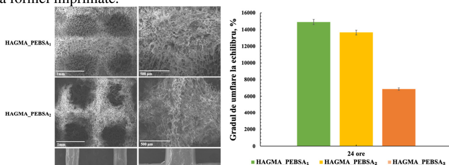
Figura 16. Morfologia hidrogelurilor și gradul de retenție al fluidelor simulate corelat cu morfologia suporturilor imprimate.
