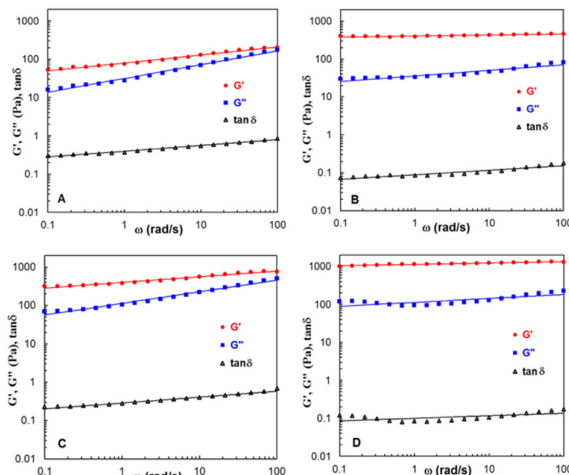
Figura 21. Parametrii vâscoelastici ai cernelurilor compozite reprezentate în funcție de frecvența de oscilație pentru \gamma = 1\% (A) L-MS1; (B) H-MS1; (C) L-MS2; (D) H-MS2.
