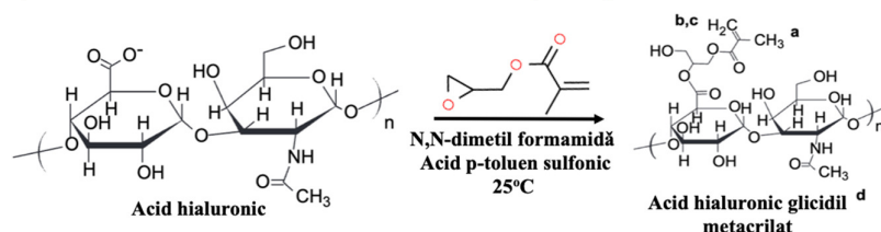
Figura 3. Reacția de funcționalizare a acidului hialuronic cu GMA [16,17].
