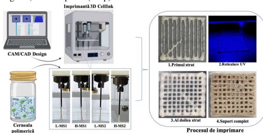
Figura 20. Prepararea matricei L/H-MS1 și L/H-MS2 foto-reticulate: 1) primul strat, 2) proces de reticulare, 3) al doilea strat, 4) matrice imprimată complet.
