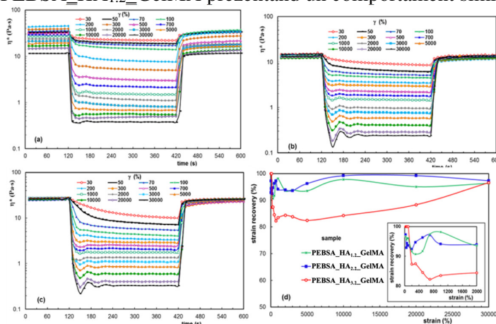
Figura 14. Comportamentul de auto-refacere a structurii după deformare, observat la gelurile reticulate (a)PEBSA_HA 1,2 _GelMA; (b)PEBSA_HA 2,2 _GelMA; (c)PEBSA_HA 3,2 _GelMA; (d) Capacitatea de recuperare în funcție de forța aplicată pentru imprimarea gelurilor. În inset se prezintă recuperarea deformării pentru \gamma \leq 2000 %.
